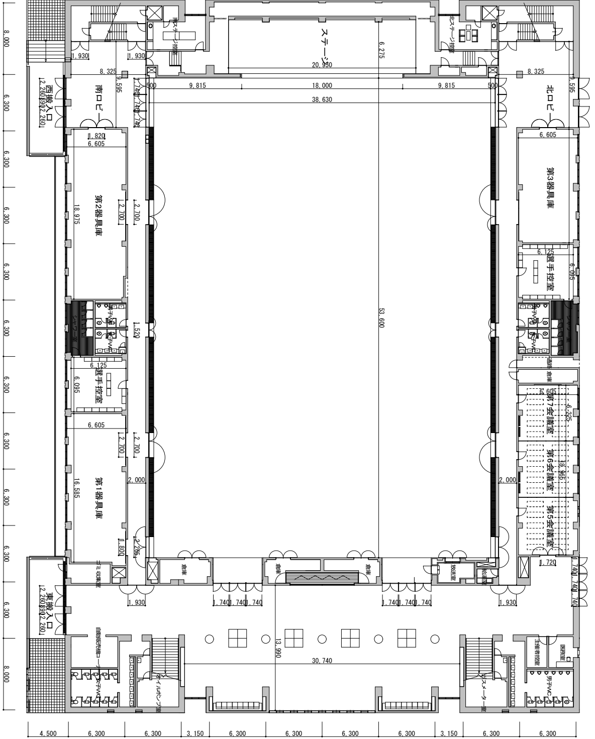
高松市総合体育館 本館1階平面図 S=1/200
